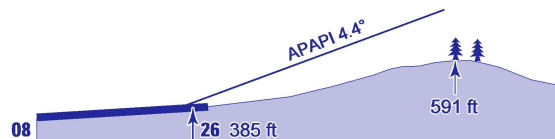
Längsprofil / Longitudinal profile: RWY 08/26
