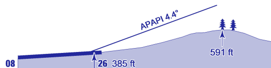
Längsprofil / Longitudinal profile: RWY 08/26
